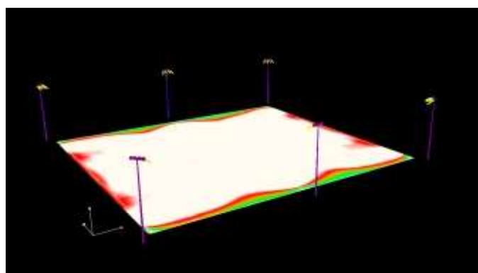
illuminamento uniforme per raggiungere lo standard del campo minimo 0.50
